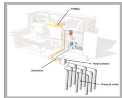
Installation sur sondes géothermiques verticales
